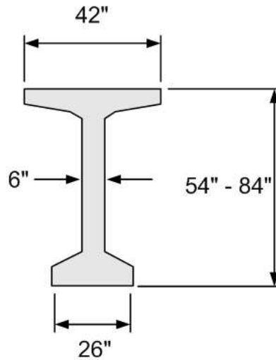
AASHTO-PCI Bulb-Tees
